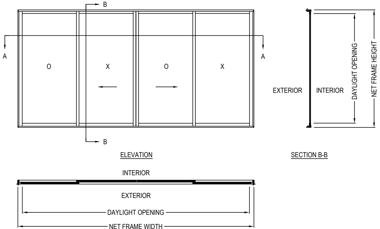
SECTION A-A
