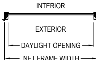
DETAIL A-A
